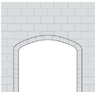
surbaissé basket handle rebajado M Flachbogen M ribassato policentrico
